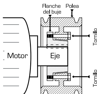
Fig 16. Montaje estándar de una polea con Buje QD
