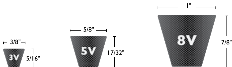
Fig 5. Sección de correas en "V" de Alta Capacidad tamaño real.
