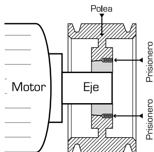
Fig 20. Instalación de una polea con Bujes Taper
